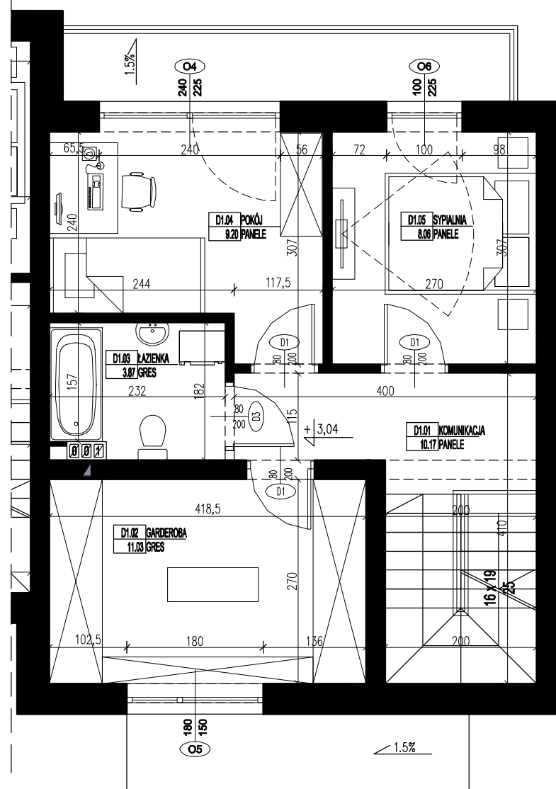
RZUT PIĘTRA LOKAL D
