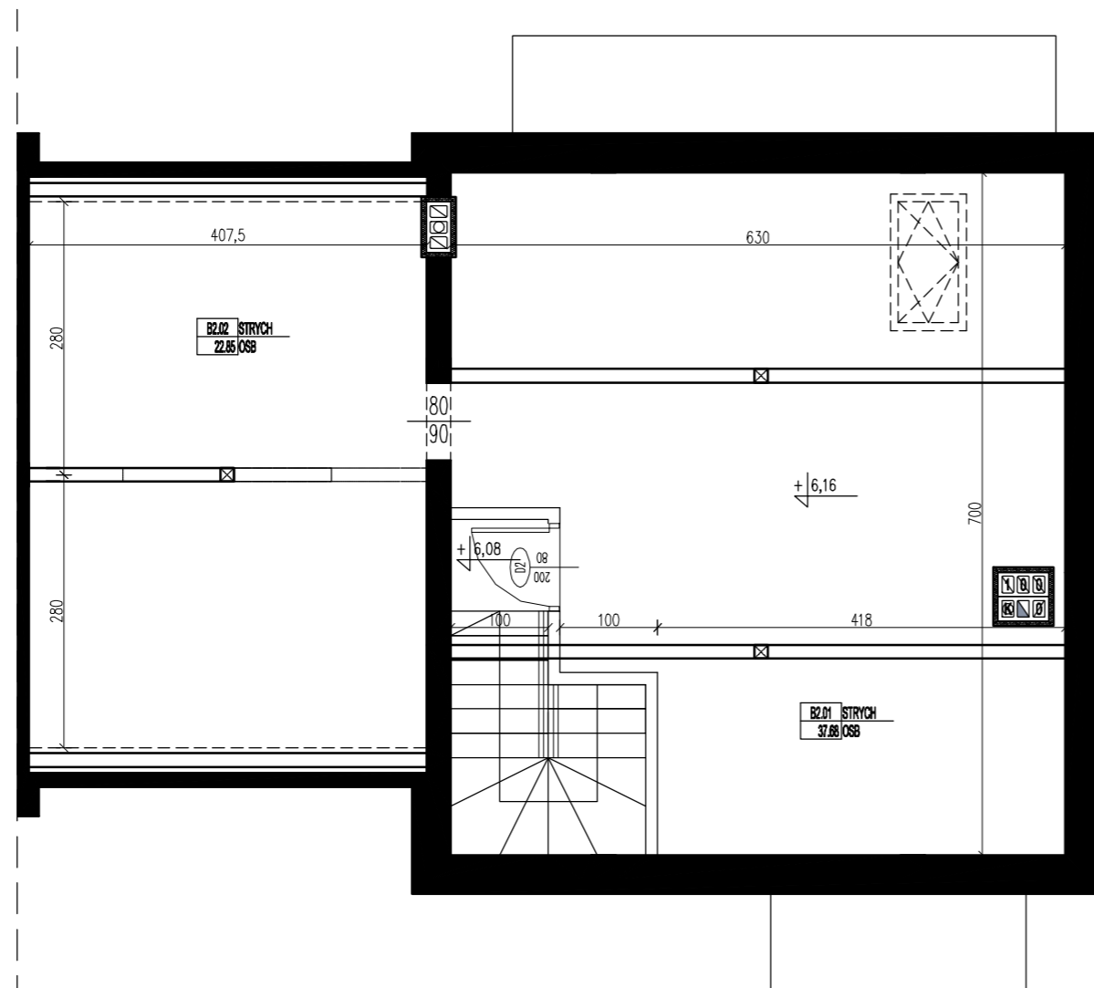
RZUT PODDASZA LOKAL B
