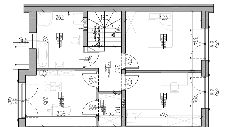
RZUT PIĘTRA
